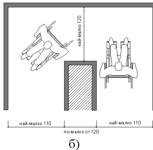
Фиг. 56. Широчина на коридора при обратен завой около препятствие
